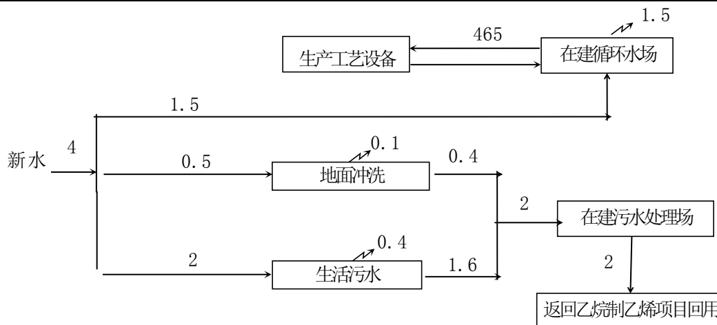
图 2.2-3 拟建工程项目水平衡图 单位： \text{m}^3/\text{h}
