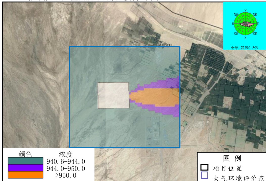
图 5.1-4 叠加现状浓度后非甲烷总烃 1 小时平均最大贡献浓度分布图单位: \mu\text{g}/\text{m}^3
