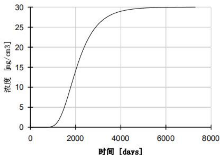
图 5.8-5 土壤底部石油类浓度-时间曲线
