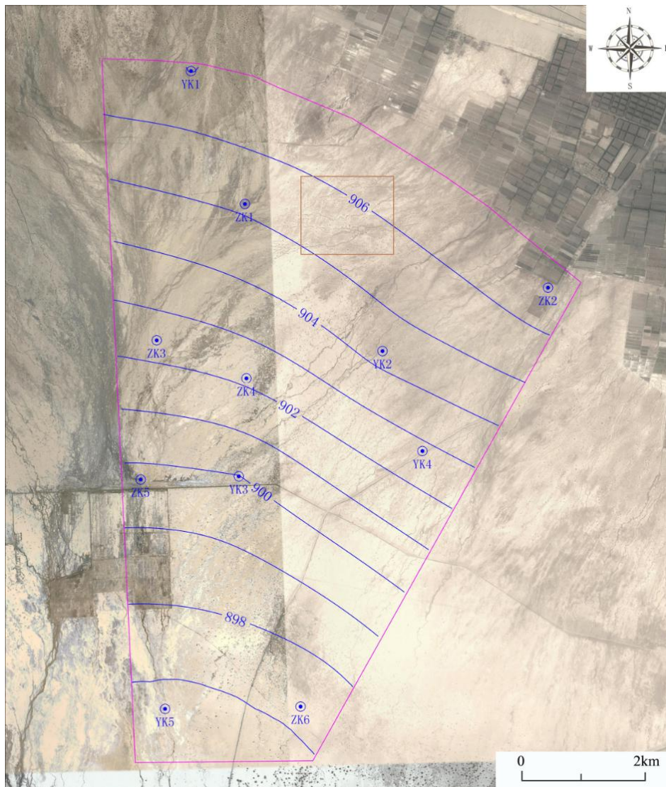
图 5.3-6 2018 年 4 月潜水初始流场图
