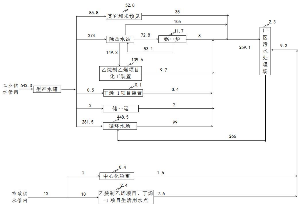
图 2.3-1 拟建工程与在建工程实施后全厂项目水平衡图 单位：m³/h
