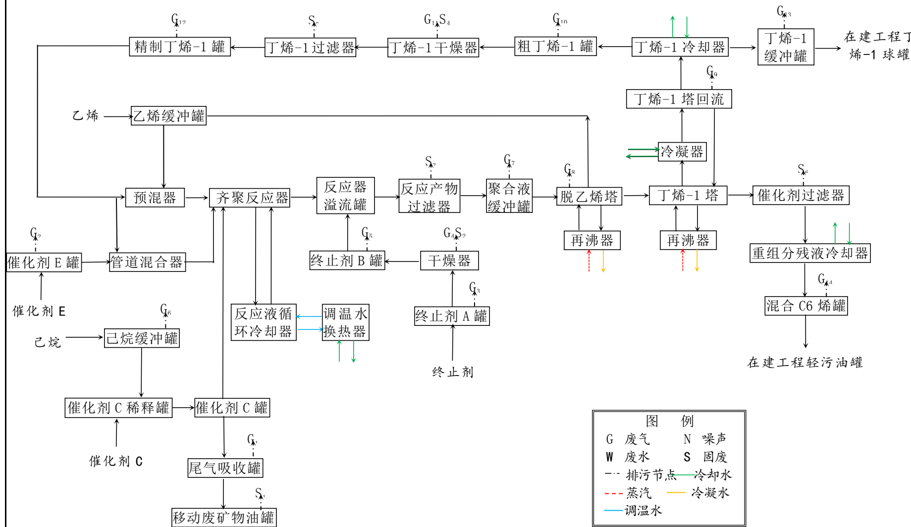
工艺流程及排污节点图
