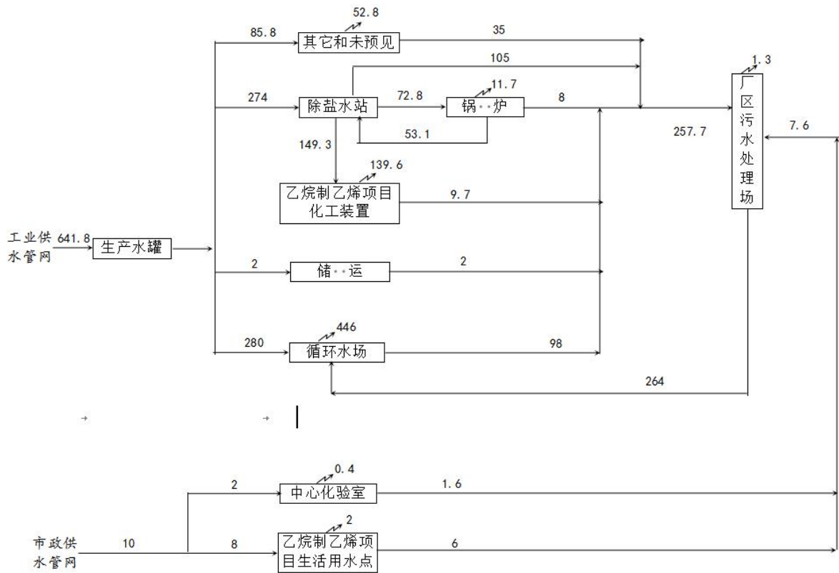
图 2.1-6 在建工程水平衡图 单位：m³/h
