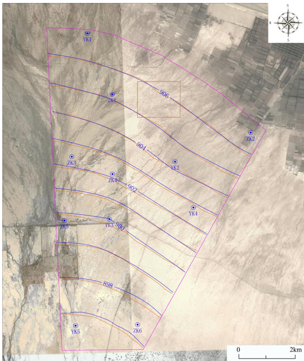
图 5.3-8 潜水含水层流场拟合图
