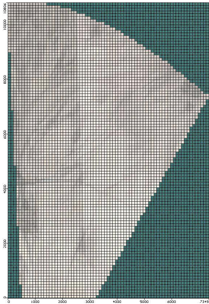
图 5.3-7 模拟区网格剖分图
