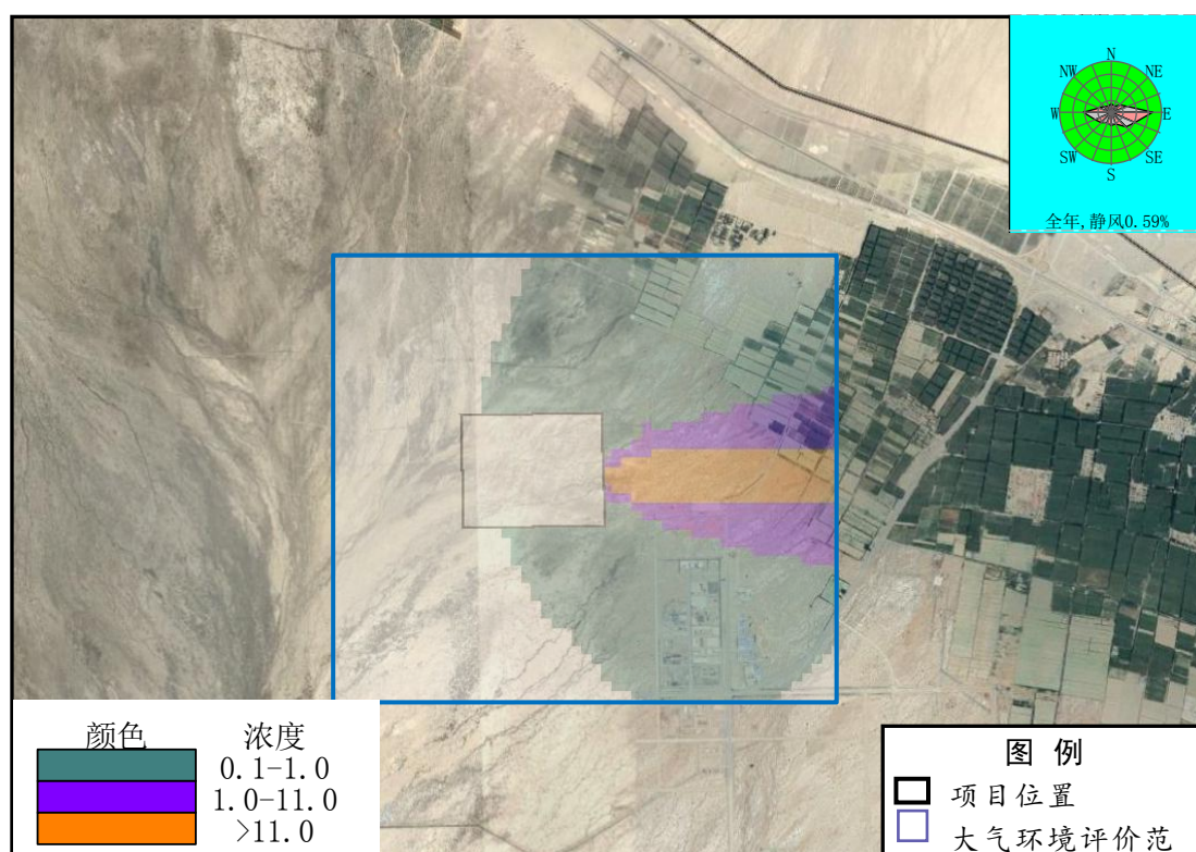
图 5.1-3 非甲烷总烃 1 小时平均最大贡献浓度分布图 单位: \mu\text{g}/\text{m}^3
