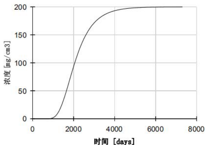
图 5.8-3 土壤底部 COD 浓度-时间曲线
