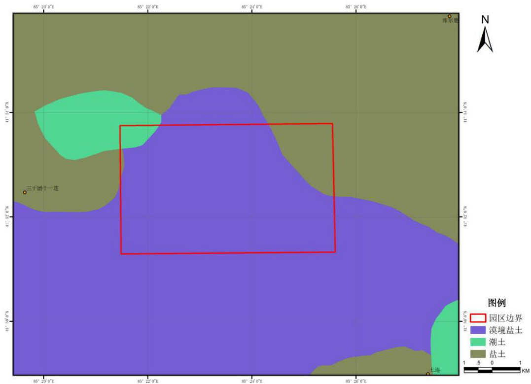
图 5.8-1 土壤类型图
