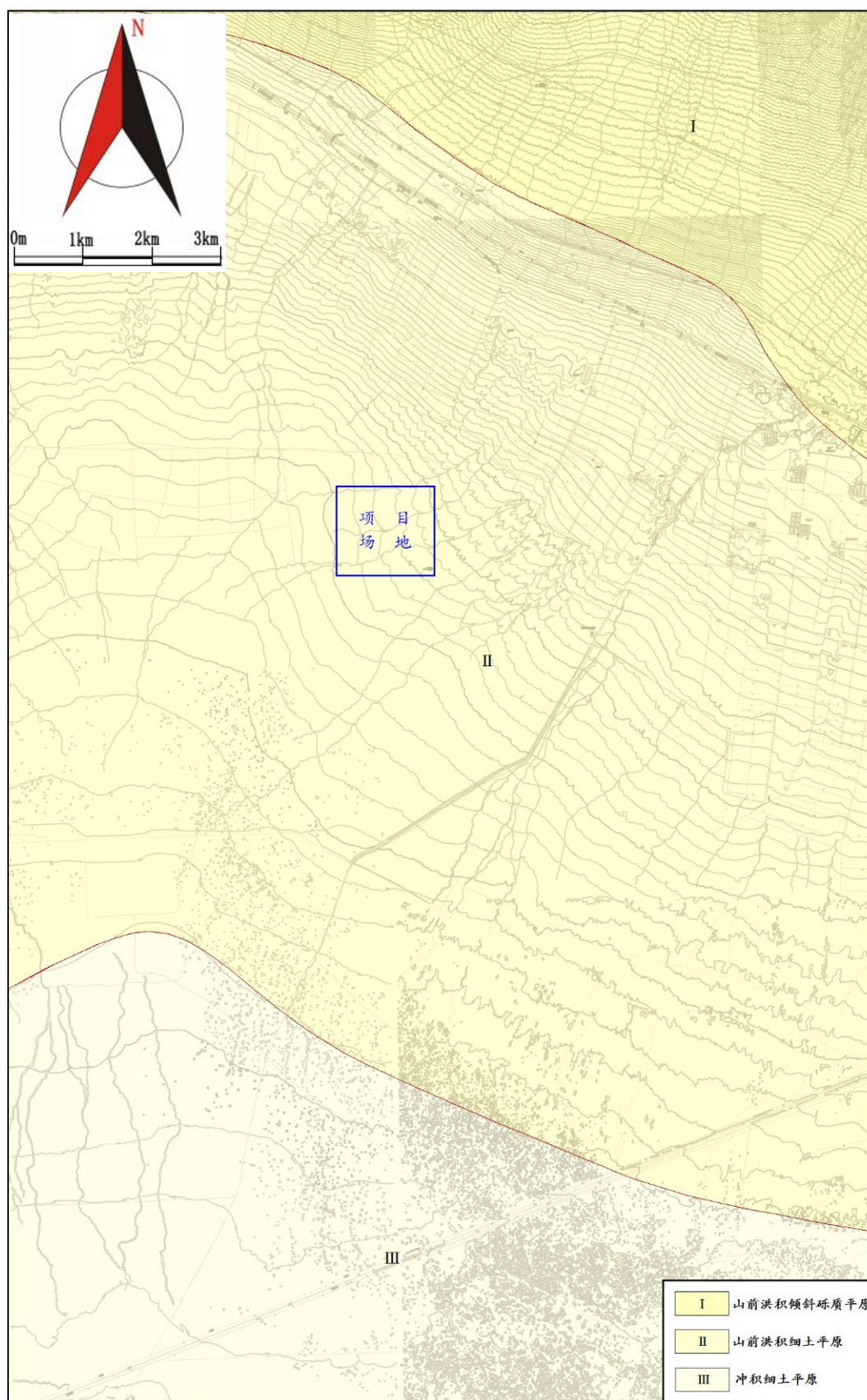
图 3.1-4 地形地貌图
