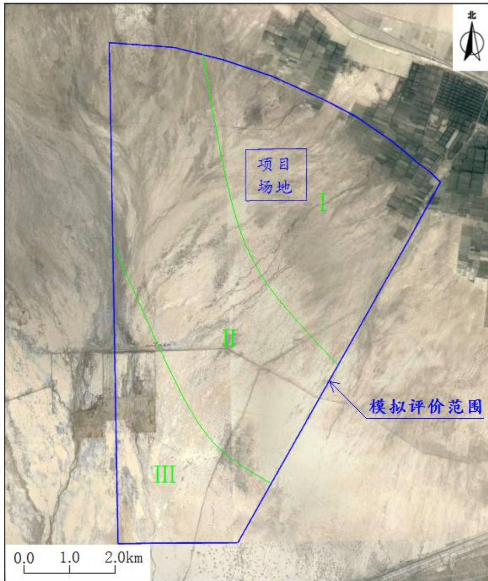
图 5.3-5 模拟区水文地质参数分区图
