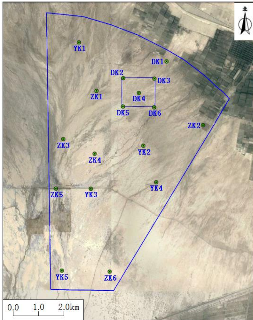
图 5.3-2 水文地质勘探孔布置图
