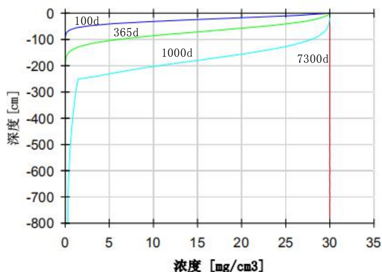
图 5.8-4 石油类在不同水平年沿土壤迁移情况
