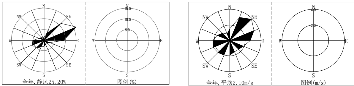
图 5.1-1 近 20 年风向及风速玫瑰图
